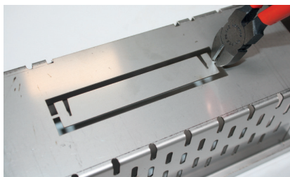
Element za učvršćenje integriran u tijelo kanala
