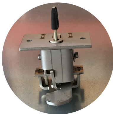
Polucilindar / ključ (LC EN 124 -A,B)
