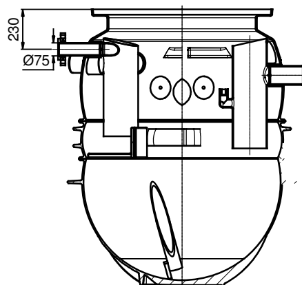
A-A ( 1:15 )
