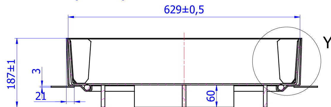
B-B ( 1 : 6 )
