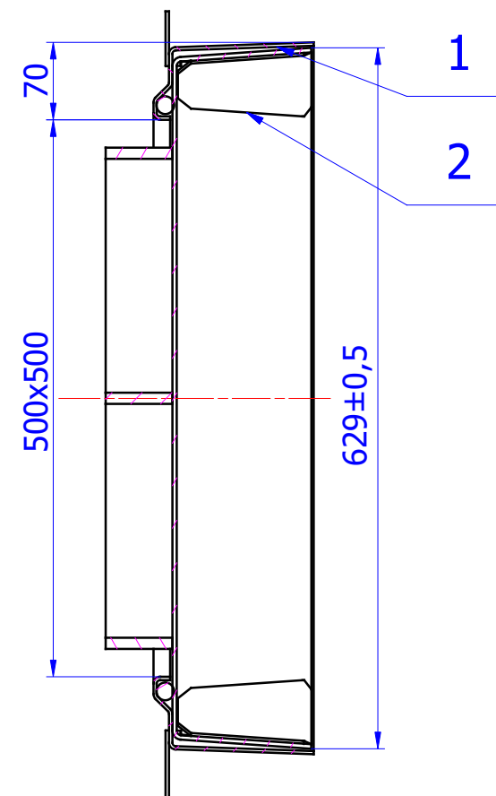
A-A ( 1 : 6 )
