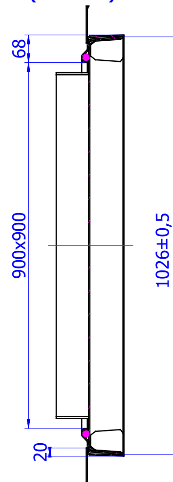
A-A (1 : 9)
