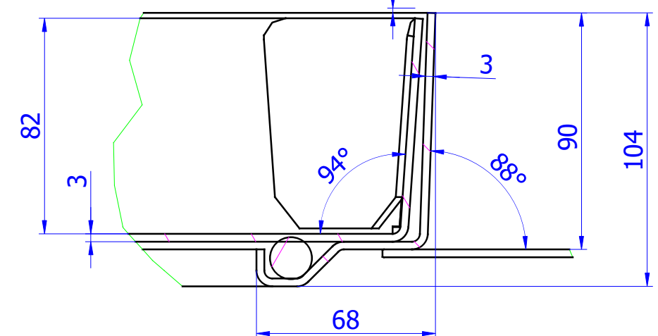
Y (1 : 2)
