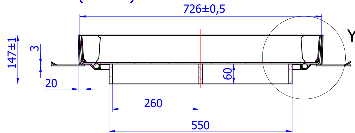
B-B ( 1 : 7 )
