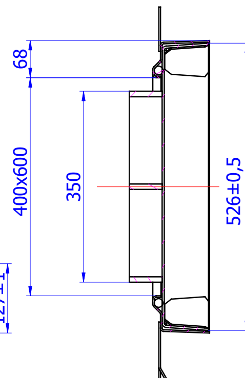
A-A ( 1 : 7 )
