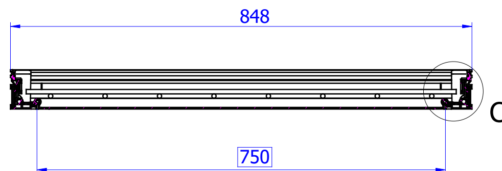
A-A ( M 1:X )
