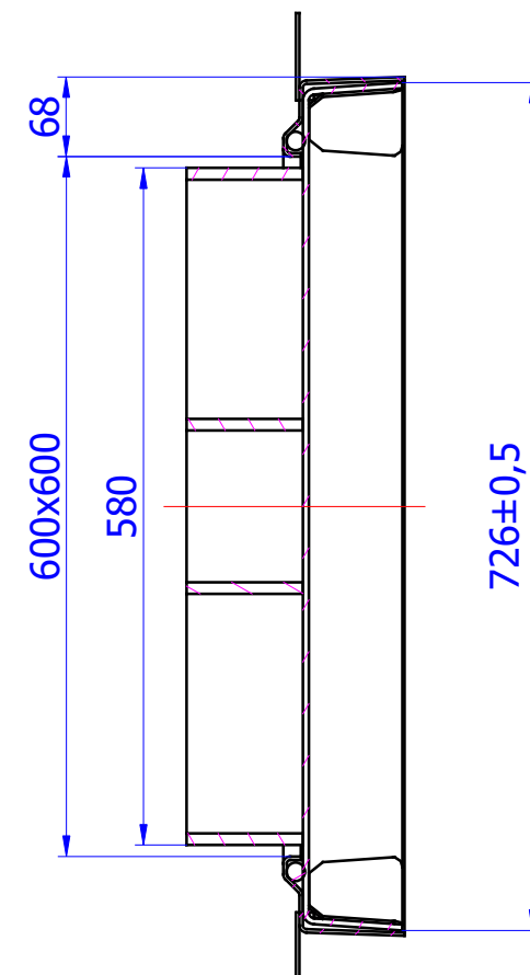
A-A ( 1 : 7 )
