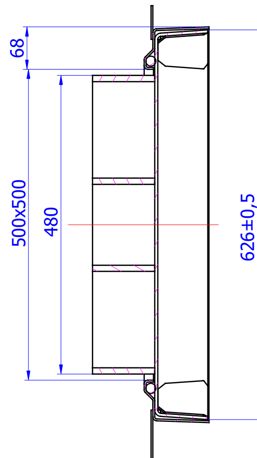
A-A ( 1 : 6 )
