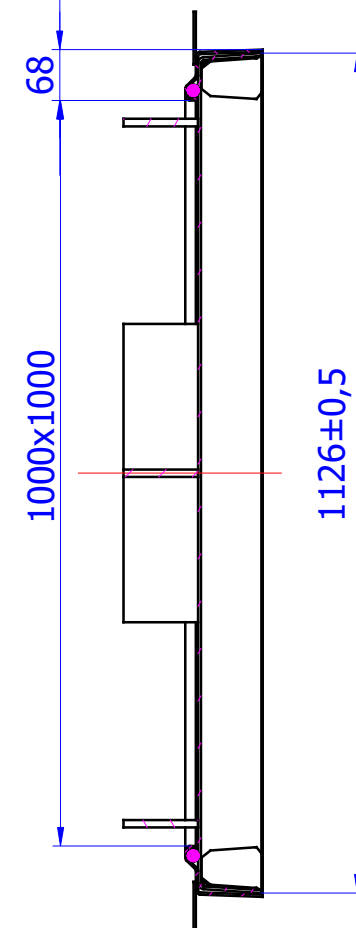
A-A ( 1 : 10 )
