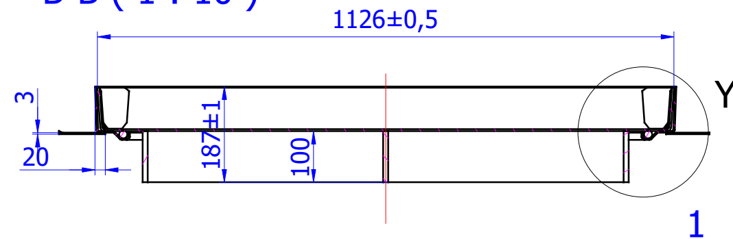
B-B ( 1 : 10 )
