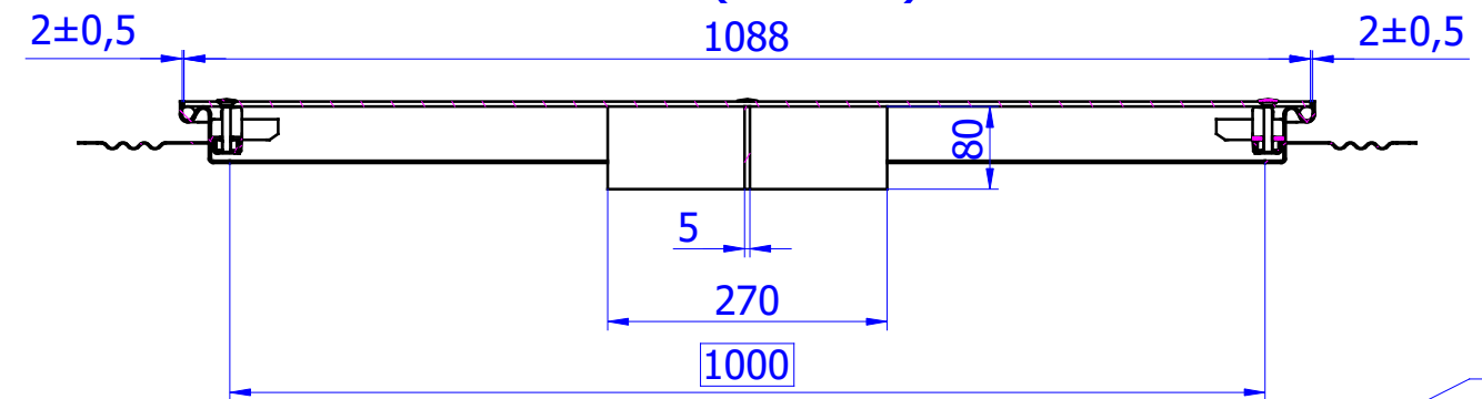
C-C ( M1:X )
