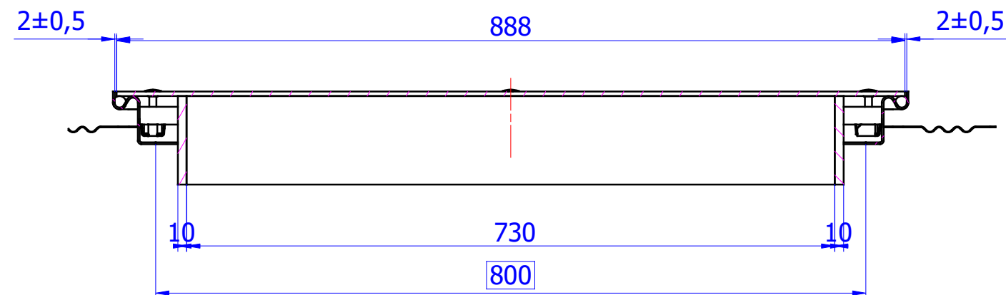
B-B ( M1:X)
