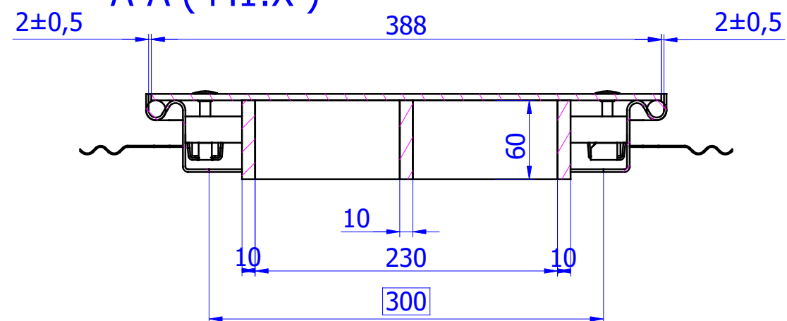
C-C ( M1:X )
