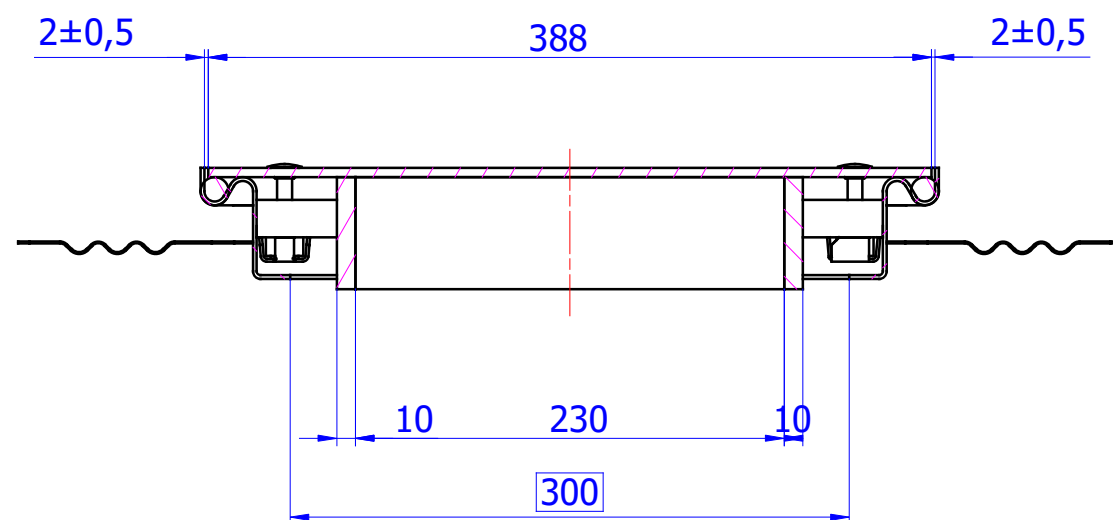
B-B ( M1:X)
