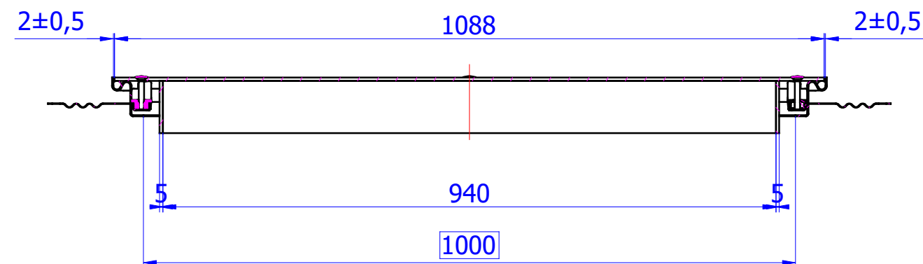
B-B ( M1:X )
