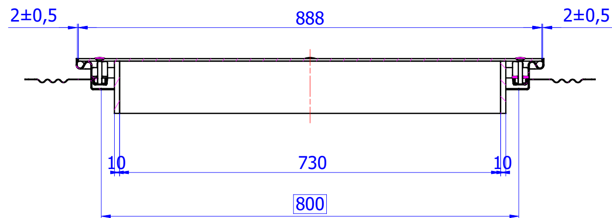
B-B ( M1:X)
