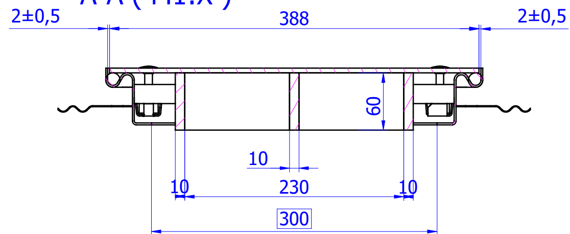
C-C ( M1:X)
