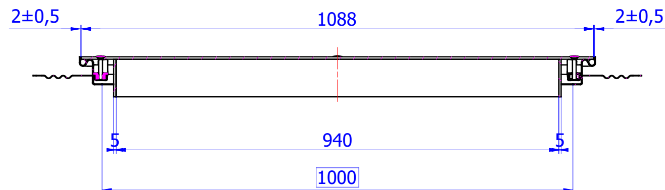
B-B ( M1:X)
