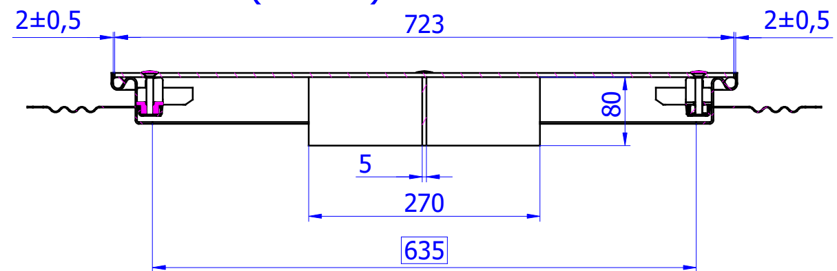
2 C-C ( M1:X)
