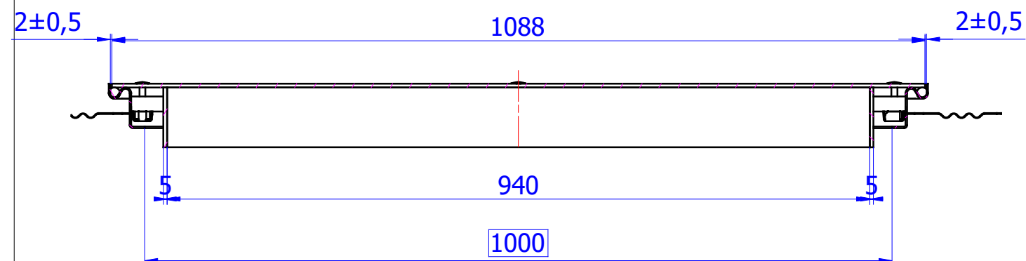
B-B ( M1:X)
