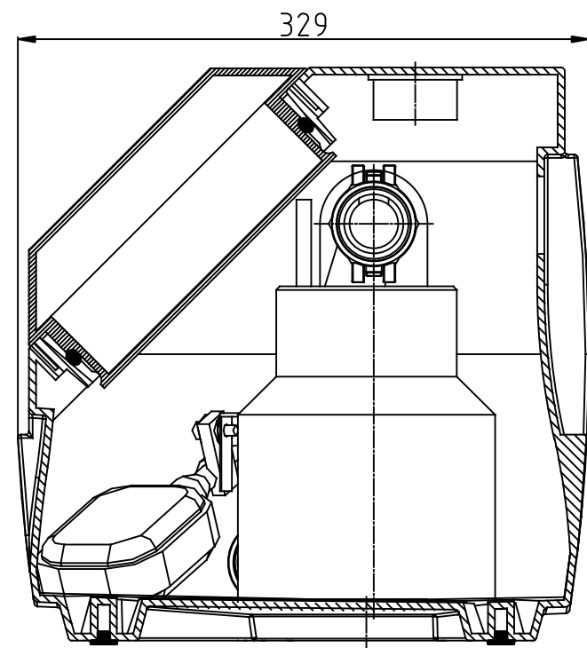
PRESJEK A-A
