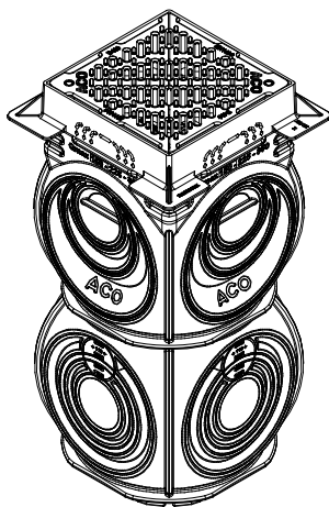
IZOMETRIJSKI PRIKAZ
