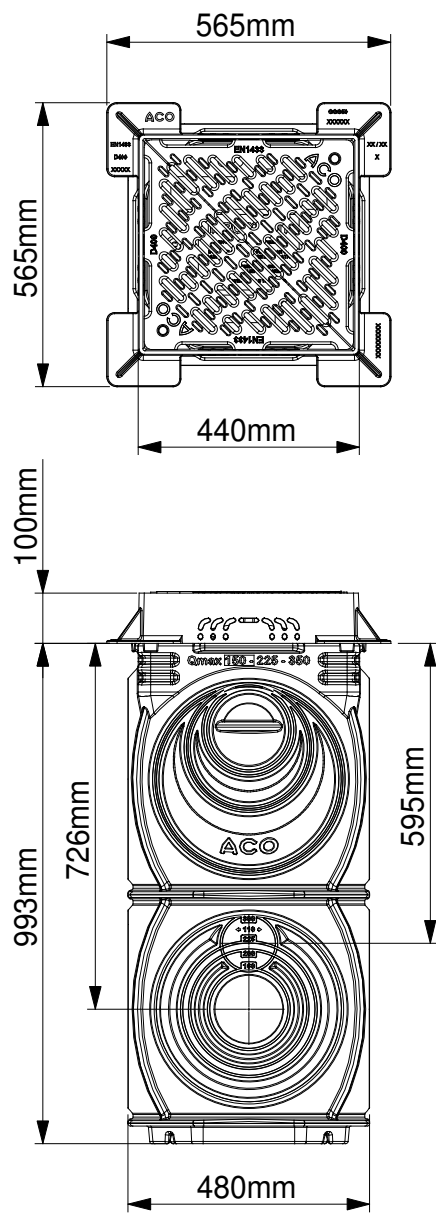
32972 - REVIZIONO OKNO ZA ULJEV/IZLJEV SA OKVIROM I POKLOPCEM D400
