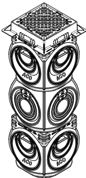
IZOMETRIJSKI PRIKAZ
