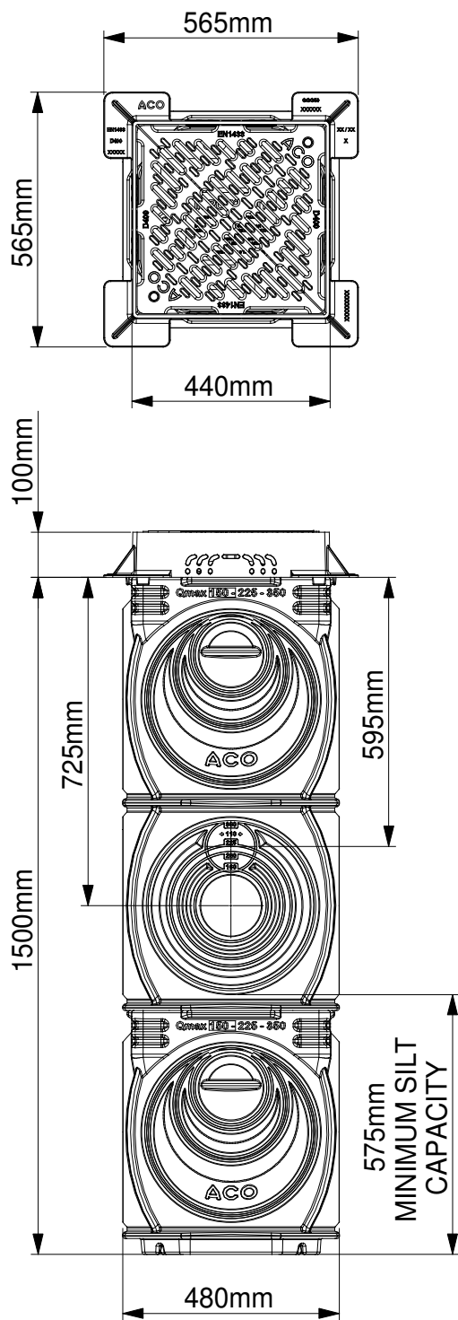
32974 - REVIZIONO OKNO ZA ULJEV/IZLJEV SA TALOŽNIKOM SA OKVIROM I POKLOPCEM D400
