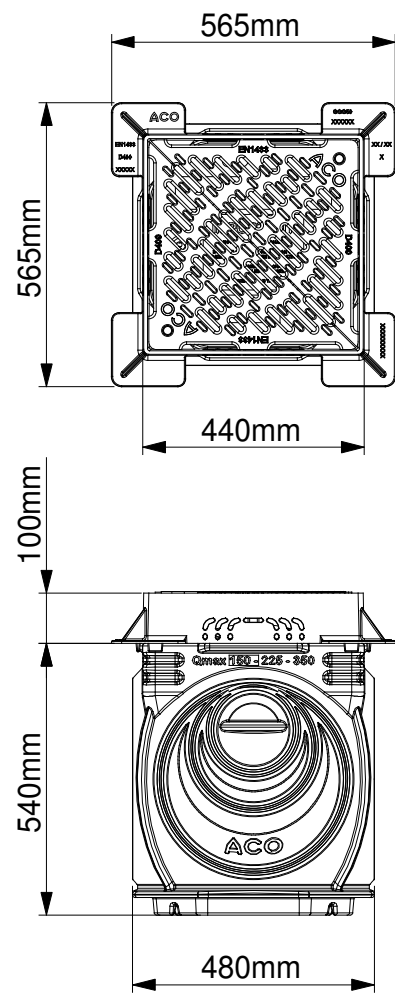
32970 - REVIZIONO OKNO SA OKVIROM I POKLOPCEM D400
