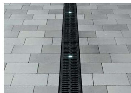
Odvodnja i ACO Eyeleds, razmak između LED 100 cm.
