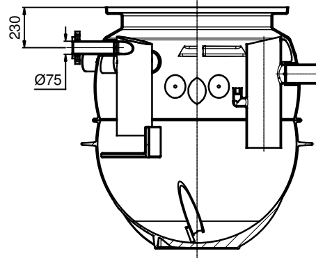
B-B ( 1 : 15 )
