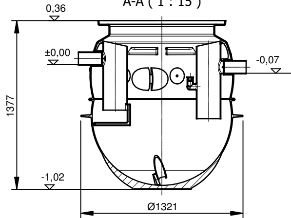
A-A ( 1 : 15 )
