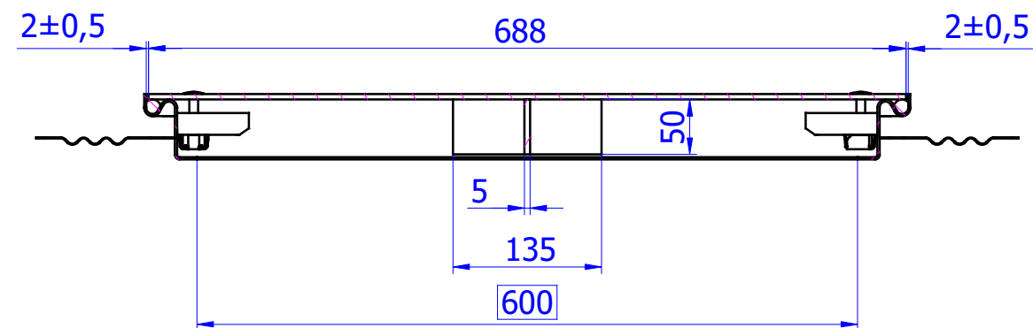
C-C ( M1:X )
