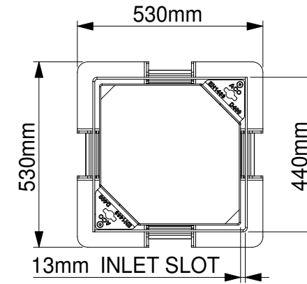
32977 - REVIZIONO OKNO ZA ULJEV/IZLJEV SA OKVIROM I POKLOPCEM D400
