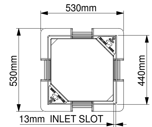
32978 - REVIZIONO OKNO ZA ULJEV/IZLJEV SA TALOŽNIKOM SA OKVIROM I POKLOPCEM D400
